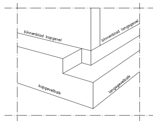
langsgevelspouw dieper dan kopgevelspouw
