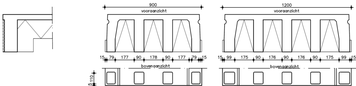
geisoleerd kopschot met oplegnokken
