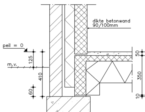
betondetail 1A
