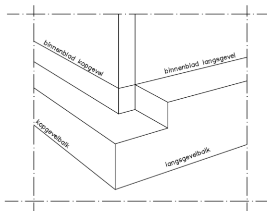
kopgevelspouw dieper dan langsgevelspouw
