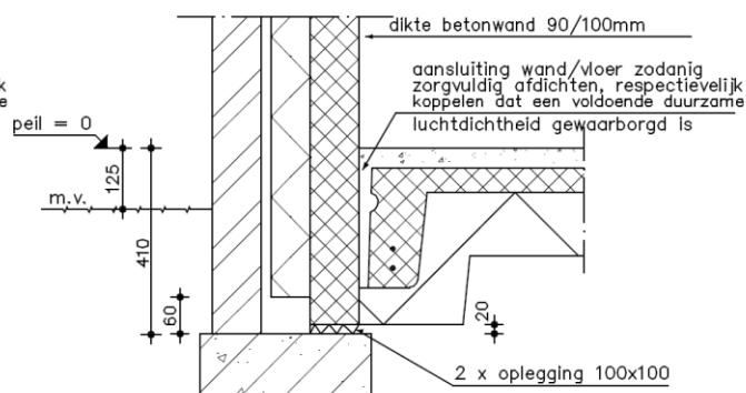
betondetail 5
