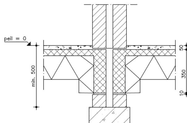
indien wand woningscheidend zie tabel 5 detail 2D
