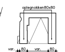
geisoleerde kop met oplegnokken
