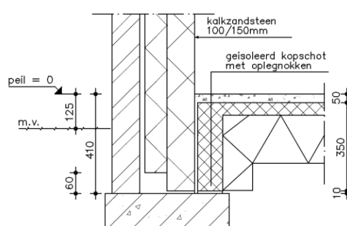
kalkzandsteendetail 1B
