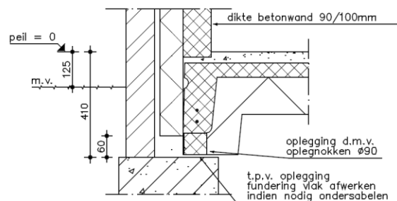
betondetail 6
