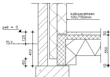
kalkzandsteendetail 1A
