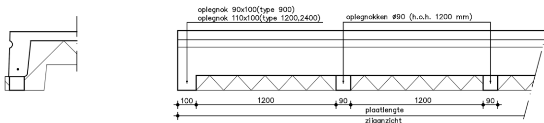
oplegnokken voorspanbalk type 900,1200 en 2400
