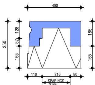
Dwarsdoorsnede Type WVR 400 Erkerplaat
