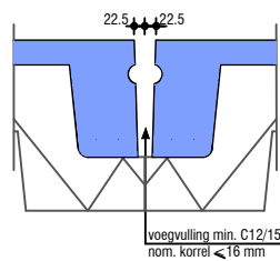
Algemeen voegdetail
