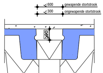
Voegdetail t.p.v. stortstrook
