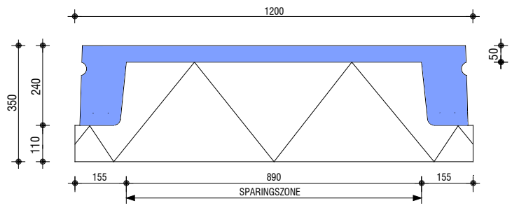
Dwarsdoorsnede Type WVR 1200
