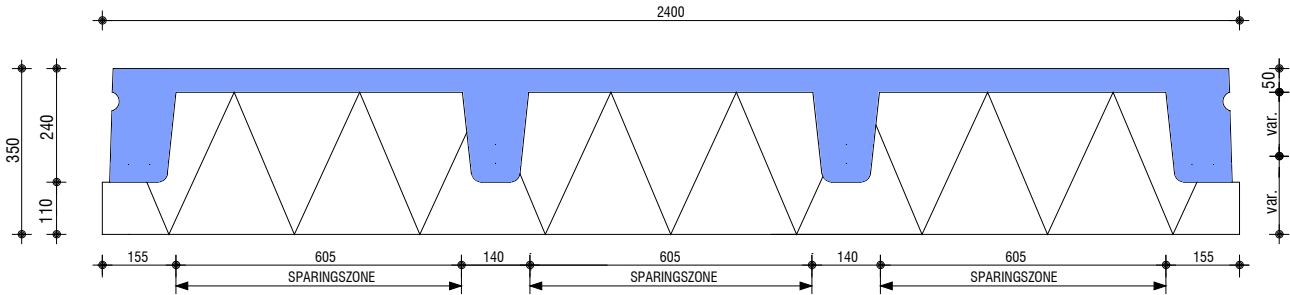
Dwarsdoorsnede Type WVR 900
