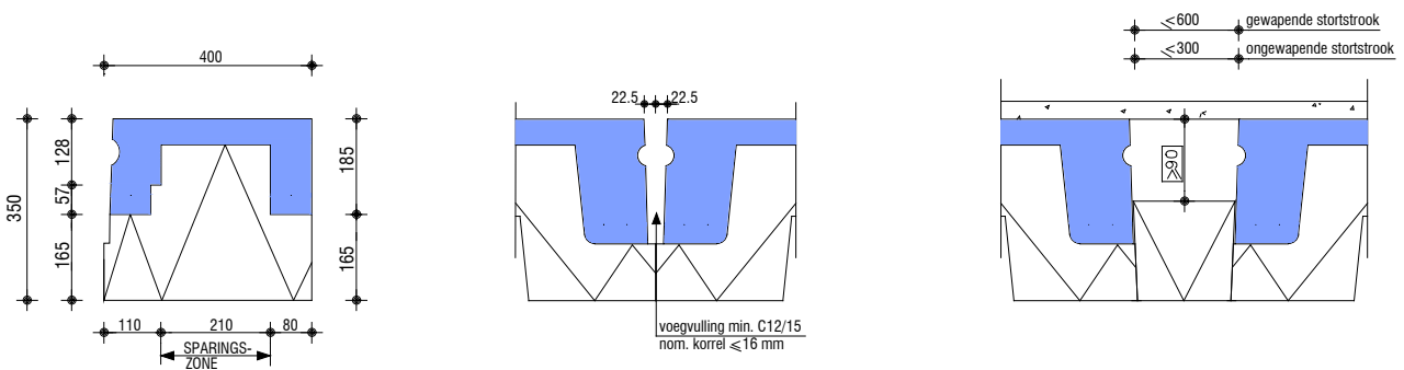
Dwarsdoorsnede Type WVR 400 Erkerplaat
