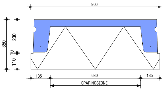
Dwarsdoorsnede Type WVR 900
