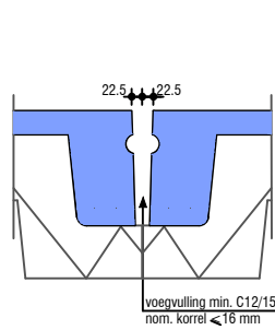
Algemeen voegdetail
